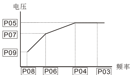
图二：任意V/F曲线设定
