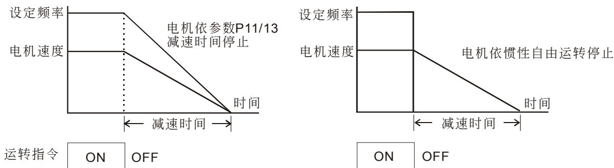
图一：减速刹车
